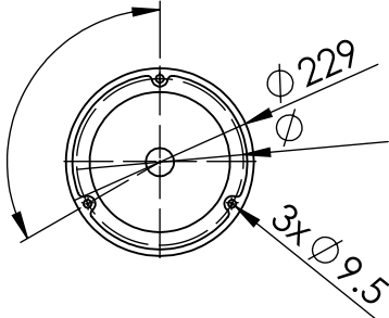
FUSSFLANSCH ELEMENT
